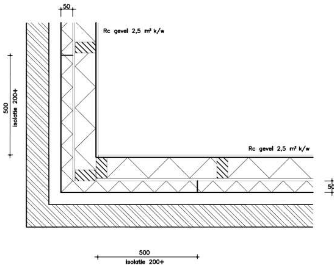
Doorsnede 2/BG
